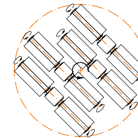
Draufsicht Rotationseinheit
